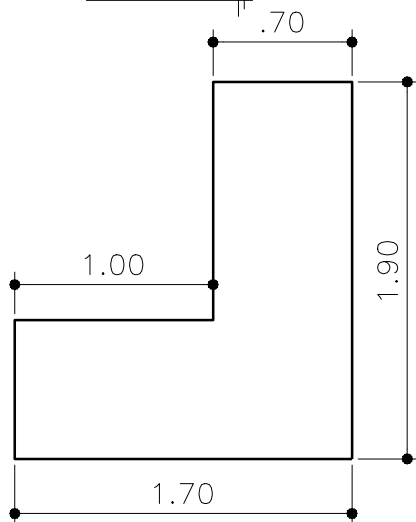
PLANTA BAIXA 1:25
