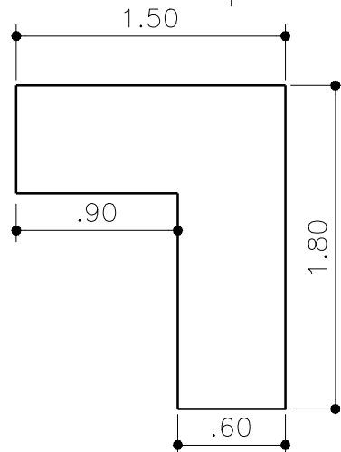
PLANTA BAIXA 1:25
