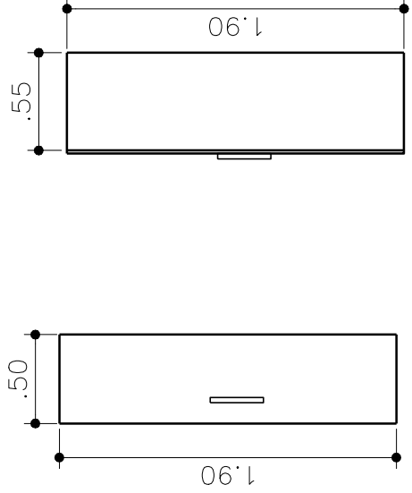
VISTA FRONTAL 1:25
