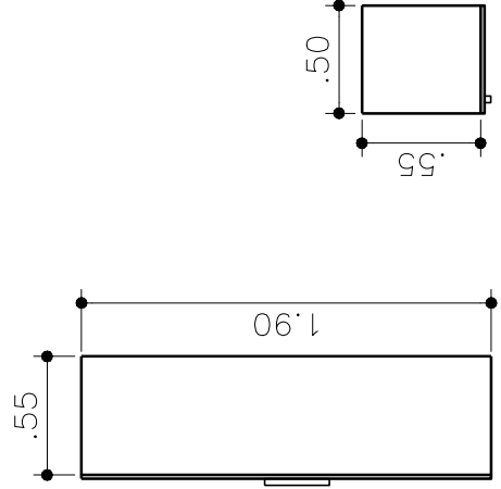
VISTA LATERAL 1:25
