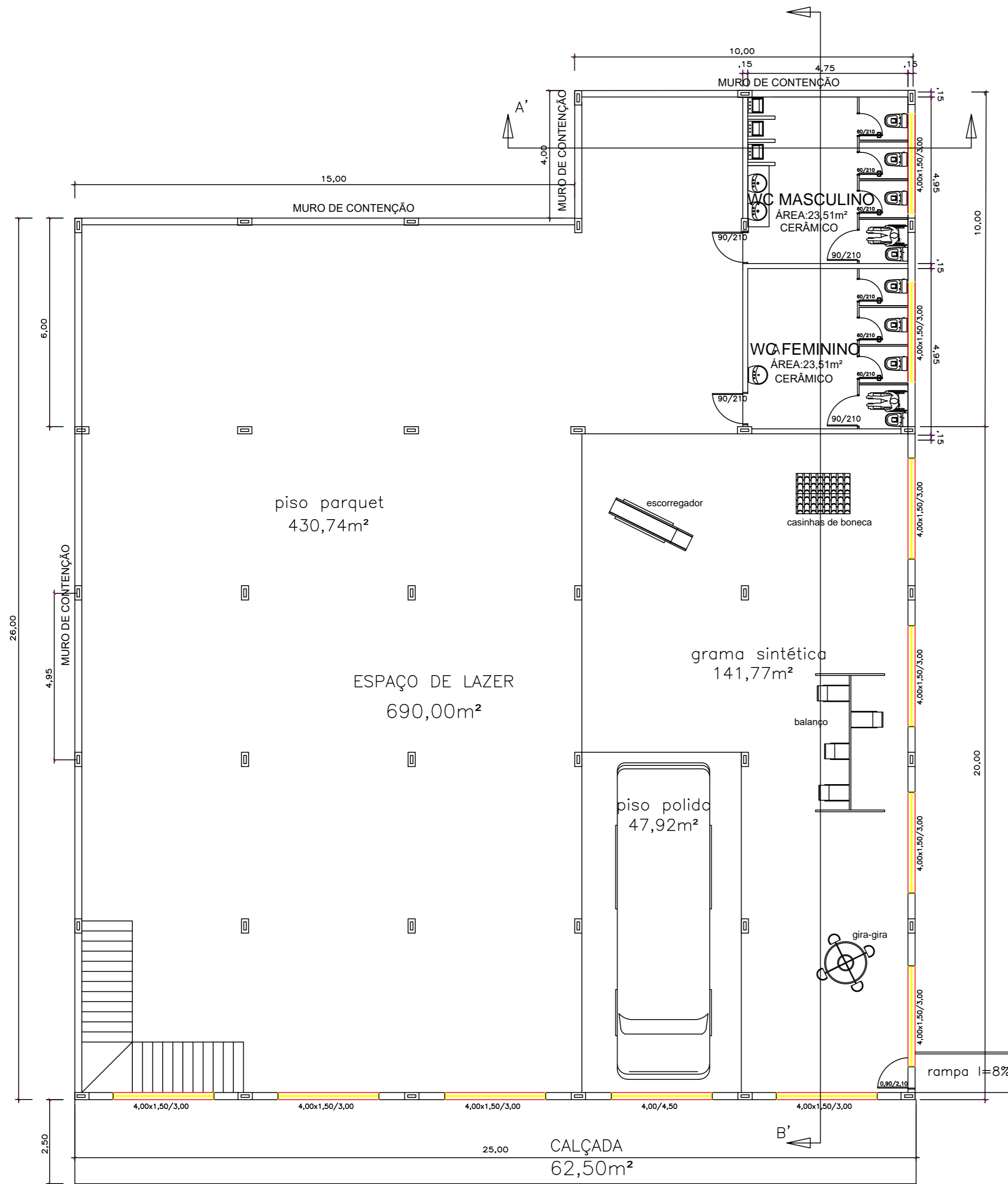
PLANTA BAIXA TÉCNICA A= 690,00m 2
